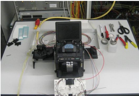
LWL spleissen
